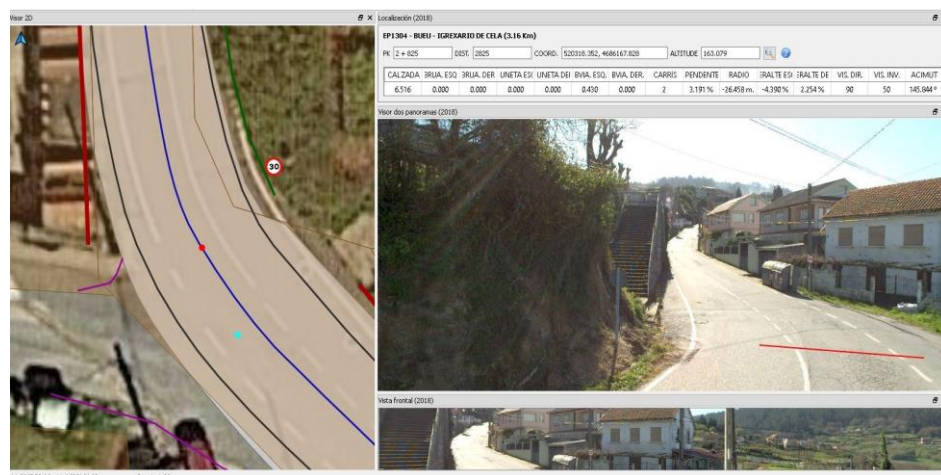
PQ 2+825 (ME)
